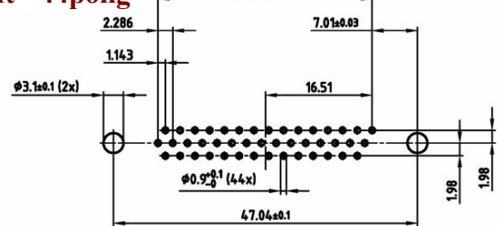
Stift - 44polig
