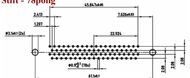
Stift - 78polig
