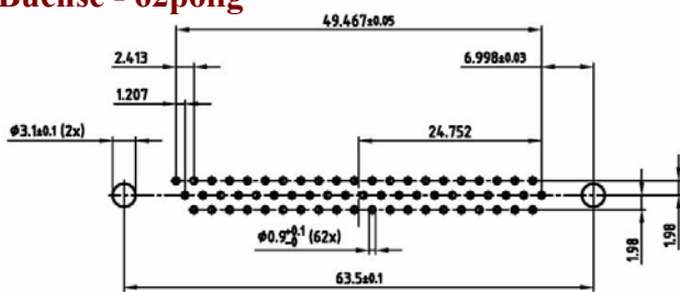
Buchse - 62polig
