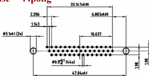
Buchse - 44polig
