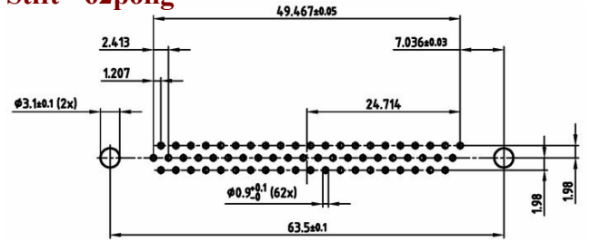
Stift - 62polig
