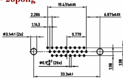
Buchse - 26polig
