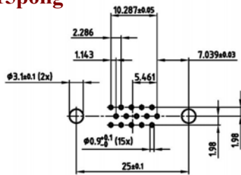
Buchse - 15polig
