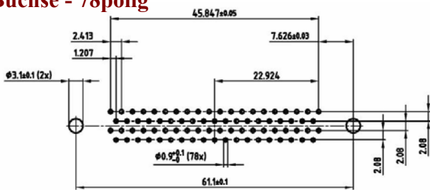
Buchse - 78polig
