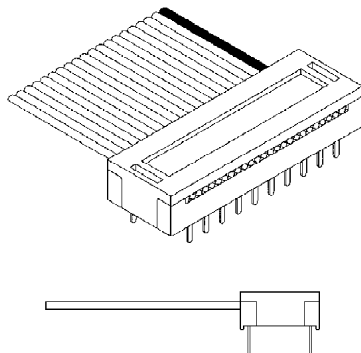
DIP-VERBINDER 0,3"
