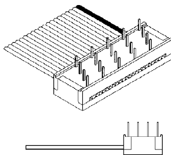
LÖTVERBINDER
