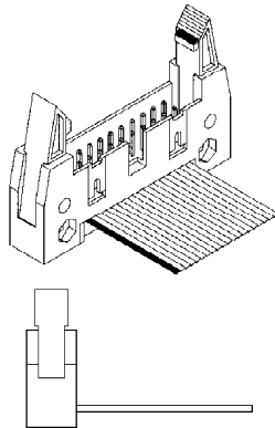
STECKERLEISTE
