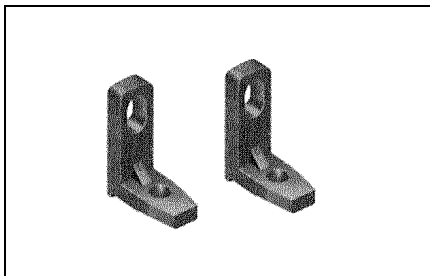
BEFESTIGUNGSWINKEL Material: Polyester GV, UL 94 V0
