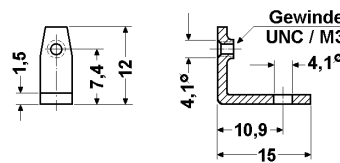
BEFESTIGUNGSWINKEL Metall • mit Gewindebohrung
