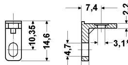
BEFESTIGUNGSWINKEL Metall • mit Gewindebohrung
