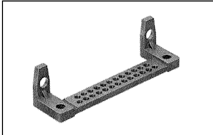
BEFESTIGUNGSWINKEL mit Mittelsteg Material: Polyester GV, UL 94 V0
