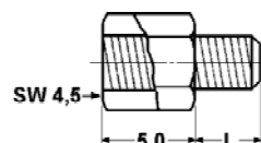
SCHRAUBVERRIEGELUNG Sechskantschraube mit Innengewinde UNC, (Schüttgut - VPE = 1 Stück)
