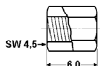
VERRIEGELUNGSSCHRAUBEN Sechskant mit Innengewinde UNC
