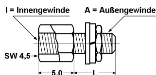
SCHRAUBVERRIEGELUNG Sechskantschraube mit Innengewinde UNC 4-40 oder M3
