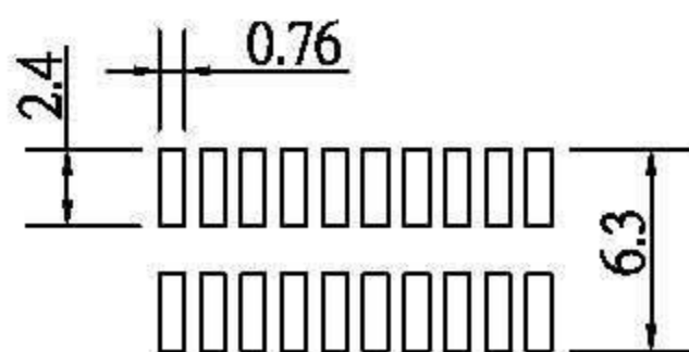
P.C.Board Layout
