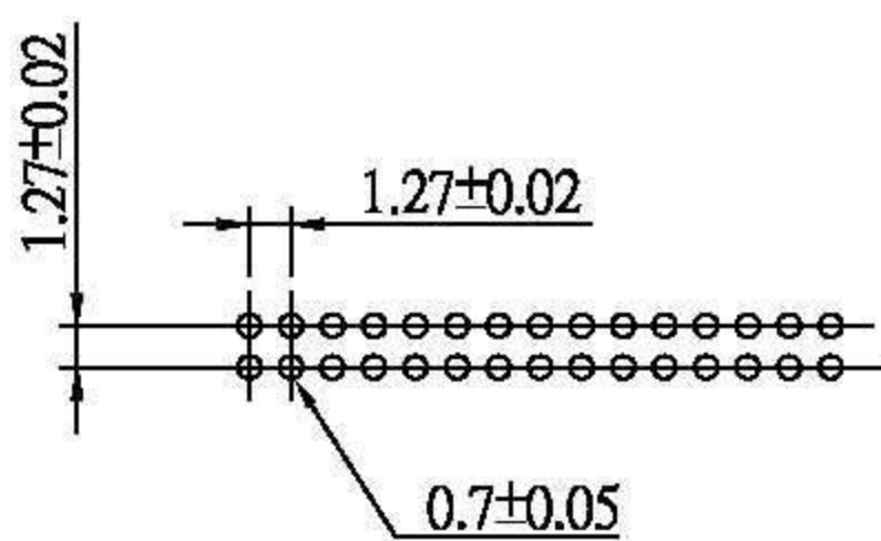
P.C.Board Layout
